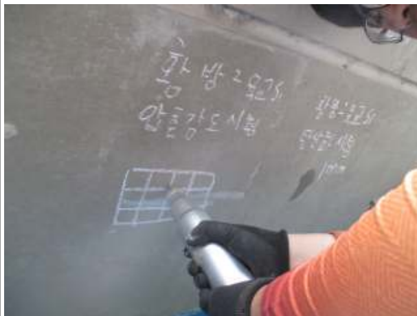
반발경도 시험
